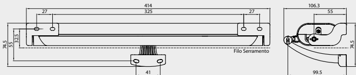
Apertura a vasistas: Ingombri e fori di fissaggio
