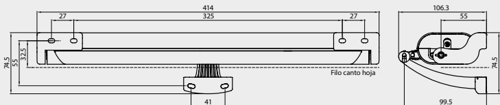
Apertura abatible: Dimensiones y agujeros de fijación
