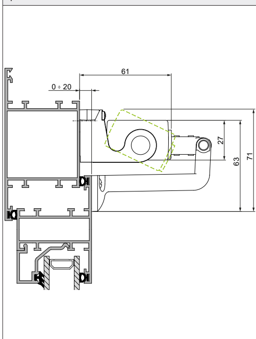
Apertura a vasistas
