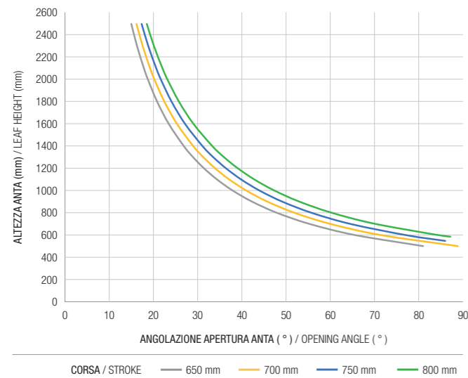
L40 Slim - 800 - Angolo di apertura anta a sporgere L40 Slim - 800 - Top hung opening angle
