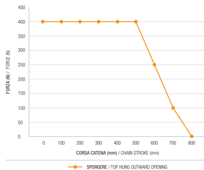
L40 Slim - 800 - Portate attuatori a sporgere L40 Slim - 800 - Actuator force - top hung and dome
